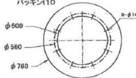
パッキン10
